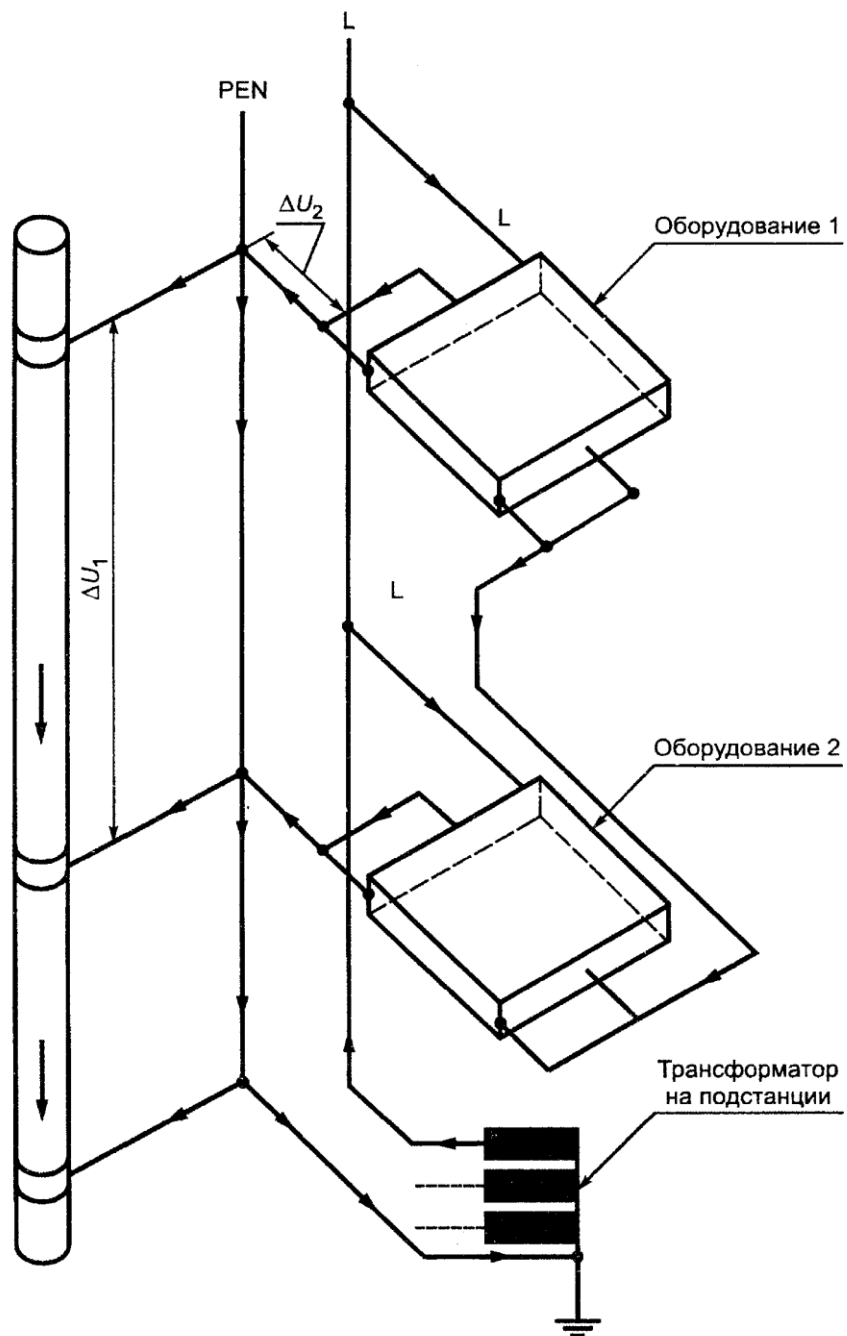
Рисунок 2а — Система заземления типа TN-C
