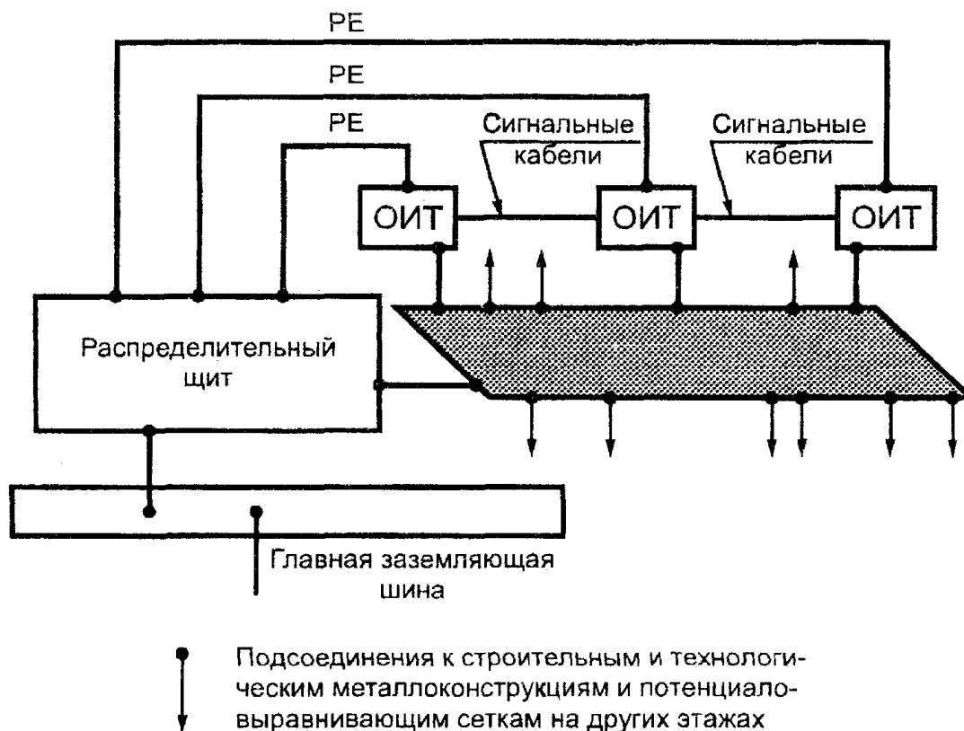
Рисунок В.3 — Система горизонтального и вертикального эквипотенциального заземления
