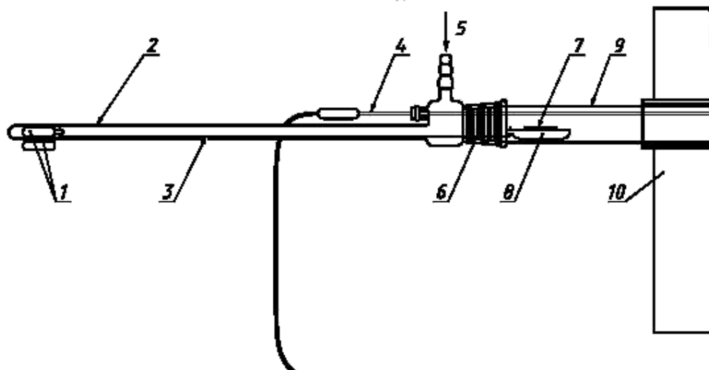
Рисунок А.1 — Устройство для ввода лодочки с образцом в трубку
