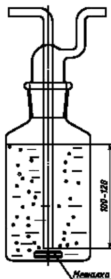
Рисунок А.2 — Пример промывочного сосуда
