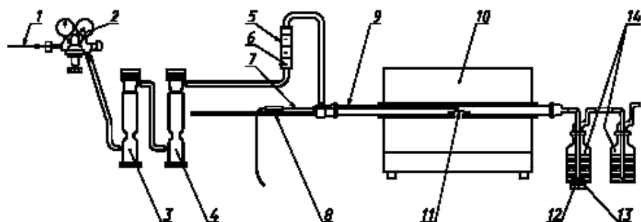
1 — сжатый воздух; 2 — редуктор; 3 — воздушный фильтр (активированный уголь); 4 — осушитель воздуха (силикагель); 5 — ротаметр; 6 — игольчатый вентиль; 7 — термометр; 8 — устройство для ввода лодочки с образцом; 9 — трубка из квар- цевого стекла; 10 — печь; 11 — лодочка с образцом; 12 — магнитная мешалка; 13 — стержень магнитной мешалки; 14 — промывочные сосуды
