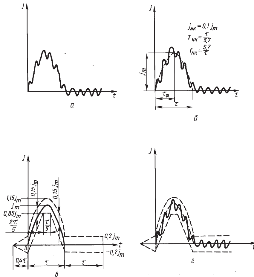
а — осциллограмма исходного импульса; б — выявление усредненного профиля импульса; в — нормированная форма импульса; г — оценка формы импульса
