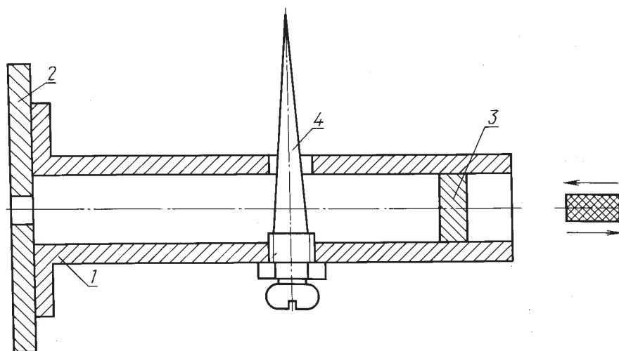
1 — волновод (10Ч23); 2 — диафрагма; 3 — поршень настройки; 4 — антенна
