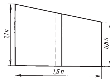
Схема реверберационной камеры
