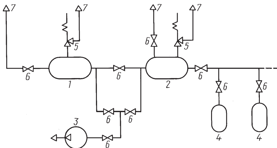
1 — камера; 2 — форкамера; 3 — вакуум-насос; 4 — емкость с газом; 5 — клапан предохранительный; 6 — запорно-регулирующая арматура; 7 — выпуск газа в атмосферу
