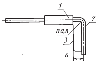
1 — изделие; 2 — вывод после изгиба; 3 — металлическая пластина для формовки
