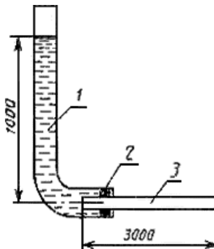
1 – вода; 2 - уплотнение; 3 - кабель
