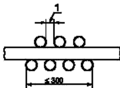
Рисунок 1 — Типичное расположение с зазором кабелей, закрепленных на обеих сторонах стандартной лестницы (категория A F/R)
