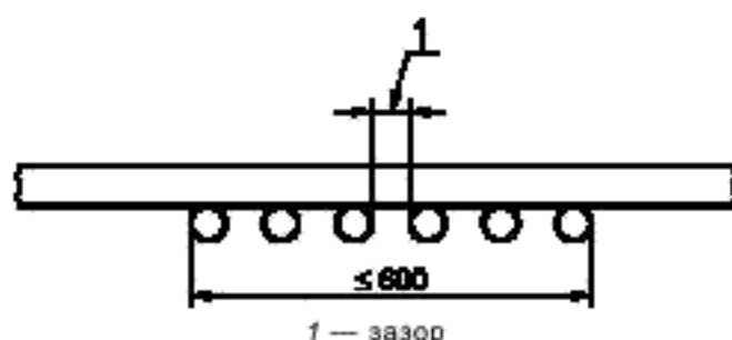
Рисунок 2 — Кабели, закрепленные на передней стороне широкой лестницы с зазором
