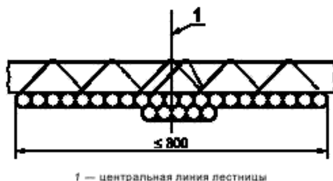
Рисунок 3 — Кабели, закрепленные на передней стороне стандартной лестницы без зазора (комплекты отрезков кабелей находятся в контакте)
