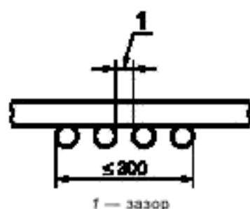
Рисунок 1 — Кабели, закрепленные на передней стороне стандартной лестницы с зазором
