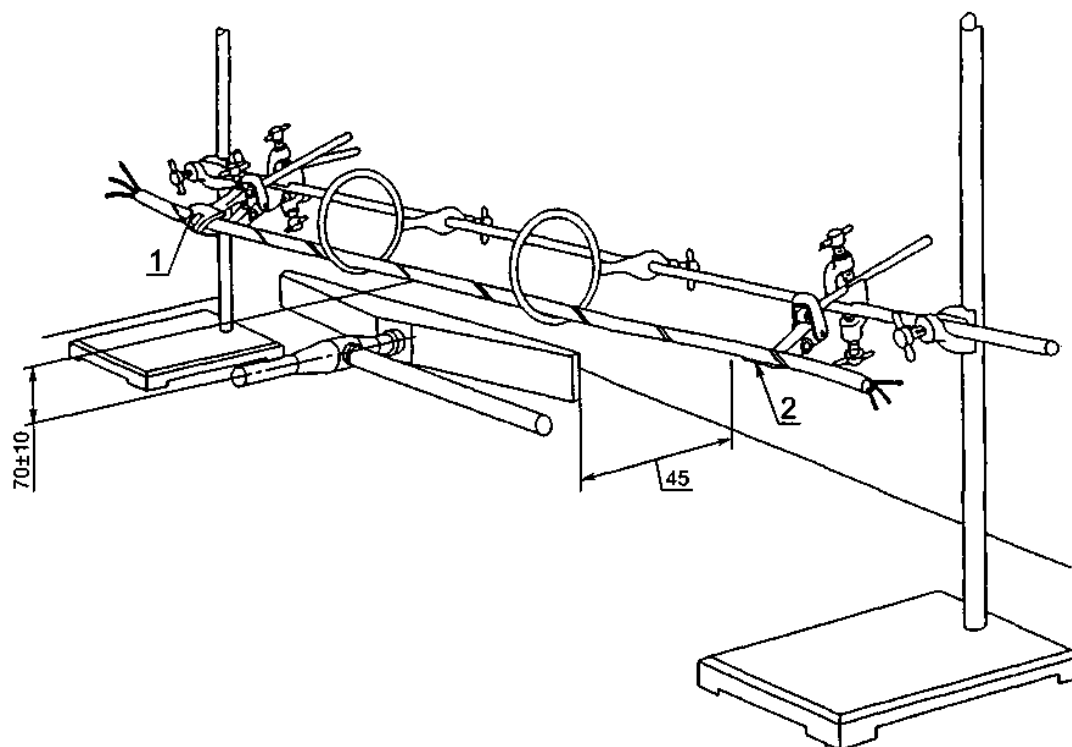
Рисунок 1 — Пример поддерживающего устройства
