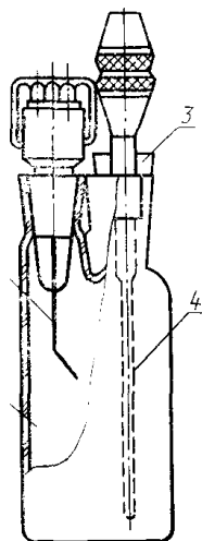
1 — реакционный сосуд; 2 — зажигающее устройство; 3 — сбросной клапан; 4 — термоэлектрический преобразователь Черт. 14
