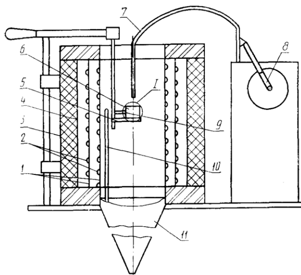
1 — стеклянные цилиндры; 2 — спиральные электронагреватели; 3 — теплоизоляционный материал; 4 — стальной экран; 5 — держатель образца; 6 — контейнер; 7 — газовая горелка; 8 — электропривод горелки; 9, 10 — термоэлектрические преобразователи; 11 — ламинатор Черт. 8
